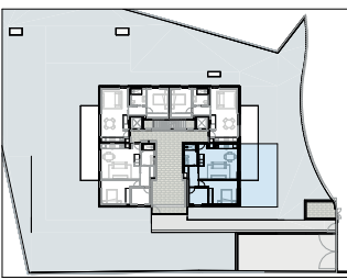
PLANTA DE LOCALIZAÇÃO piso 1
