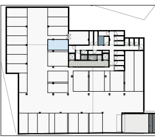
PLANTA DA GARAGEM piso -1
