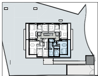
PLANTA DE LOCALIZAÇÃO piso 4
